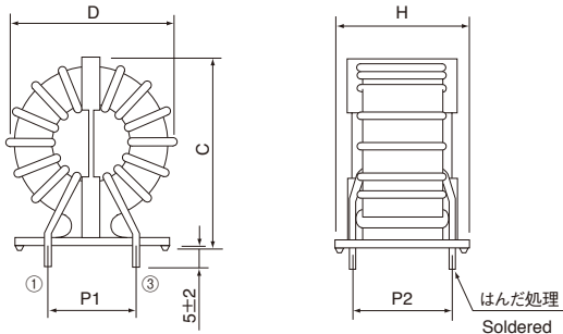
外形寸法図 (mm) DIMENSIONS (mm)
