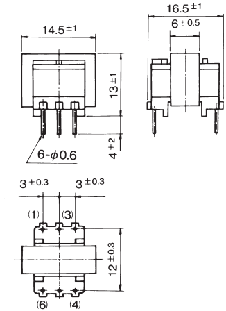
寸法図 DIMENSIONS (mm)
